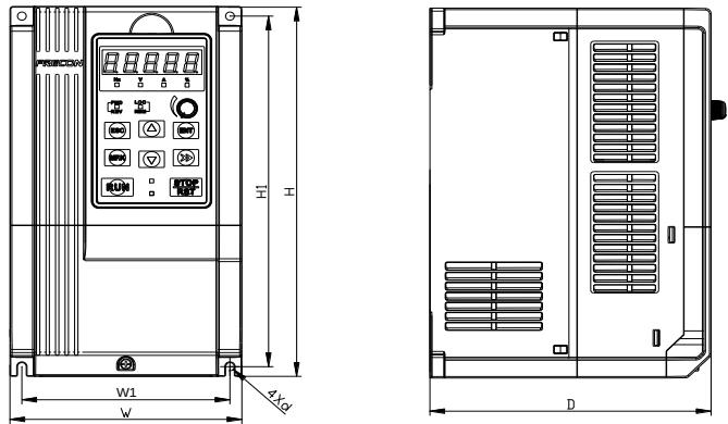
图 1-4 4~22kW 壁挂安装示意图
