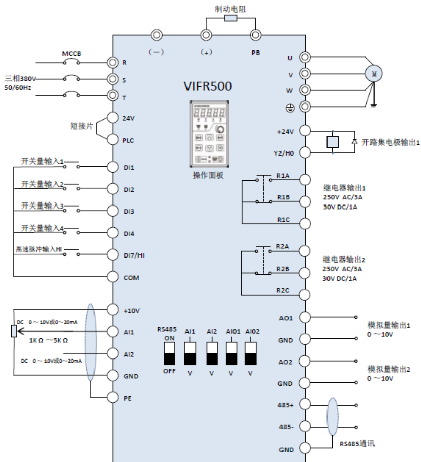
图 1-6 VIFR500 变频器接线示意图
