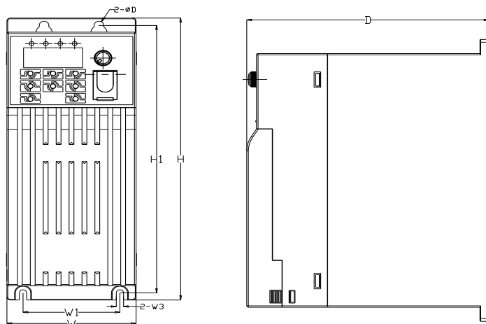
图 1-3 0.7~2.2kW 壁挂安装示意图
