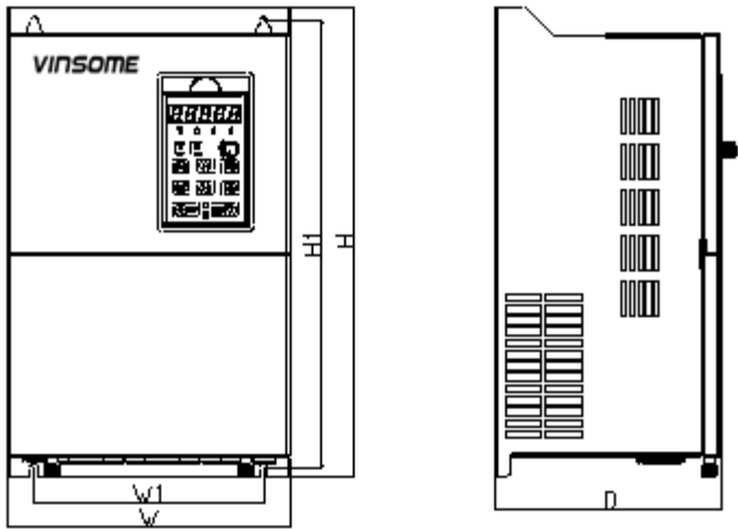
图 1-5 30~355kW 壁挂安装示意图
