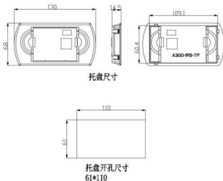
图 2-8.1 小号外引键盘带托盘安装尺寸图(VIF350(S)系列 4T:380V 2.2kW 以下标配小号外引键盘, VIF350(N)系列 4T:380V 5.5kW 以下标配小号外引键盘)
