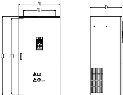
图 2-5. VIF350(S)系列 15~132KW 钣金机箱外形尺寸及安装尺寸示意图
