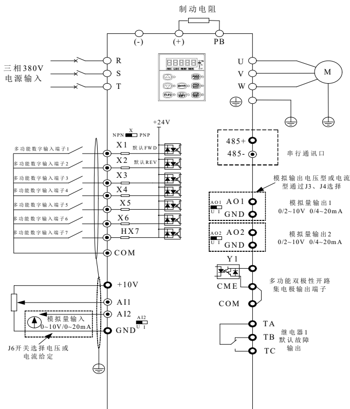
图 3-2. VIF350(S)系列 4.0~ 30kW (4T:380V 4.0 ~ 30kW), VIF350(N)系列 7.5~ 30kW (4T:380V 7.5 ~ 30kW) 三相变频器接线图
