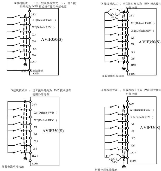
图 3-11. 四种不同模式下数字输入端子接线图
