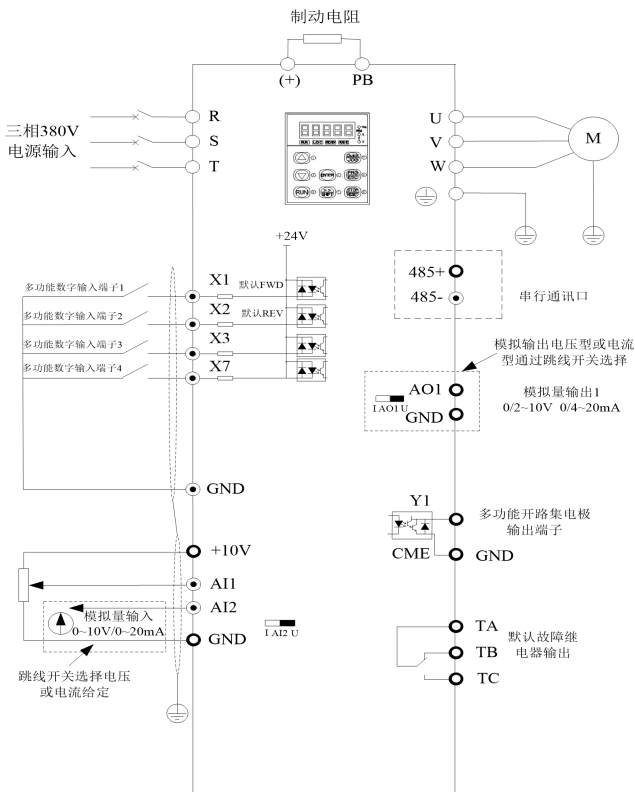
图 3-1. VIF350(S)系列 2.2kW (4T:380V 2.2 kW) 以下, VIF350(N)系列 5.5kW (4T:380V 5.5 kW) 以下三相变频器接线图
