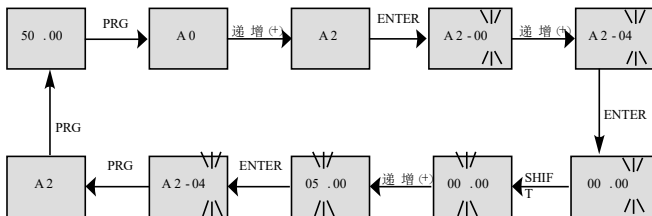
图 4-3. 参数设定操作流程
