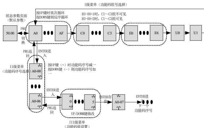
图 4.2. 三级菜单操作流程图
