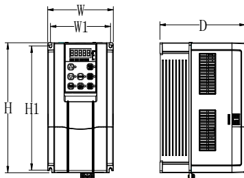
图 2-4. VIF350(S)系列 11KW 以下塑胶外形尺寸及安装尺寸示意图 (VIF350(N) 22KW 以下为塑壳机箱)
