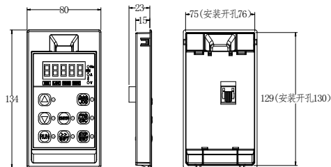
图 2-8.3 大号外引键盘带托盘安装尺寸图 (VIF350(S)系列 4T:380V 55kW 以上标配大号外引键盘, VIF350(N)系列 4T:380V 15~22Kw, 55Kw 以上标配大号外引键盘)
