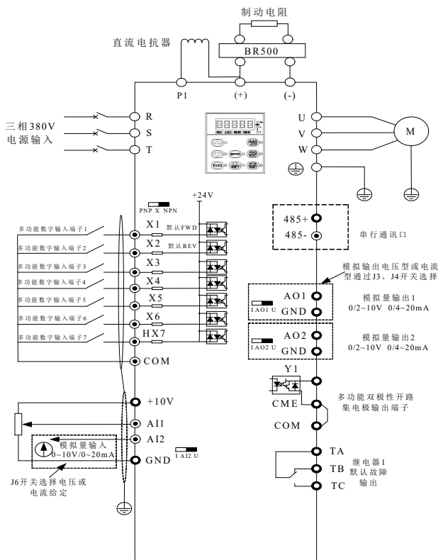
图 3-4.93Kw (4T:380V 93 Kw) 及以上三相变频器
