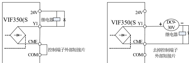
外部供电接线图
