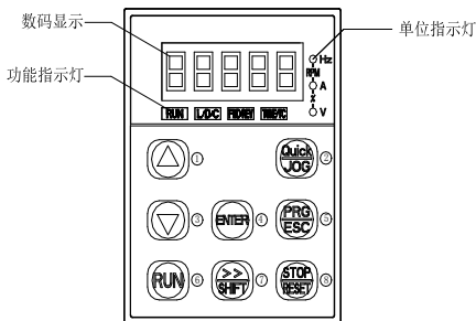
图 4-1.操作面板示意图 1 (标准配置 LED 键盘 1)
