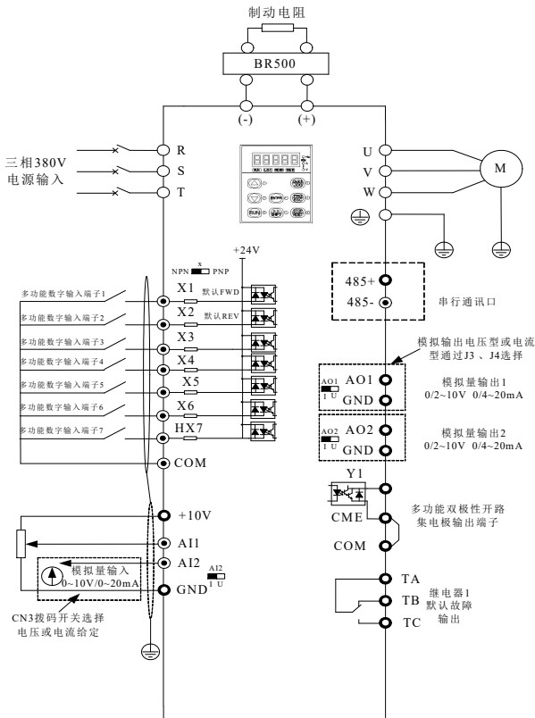
图 3-3.37~75Kw (4T:380V 37~75 Kw) 三相变频器不带制动单元功能接线图
