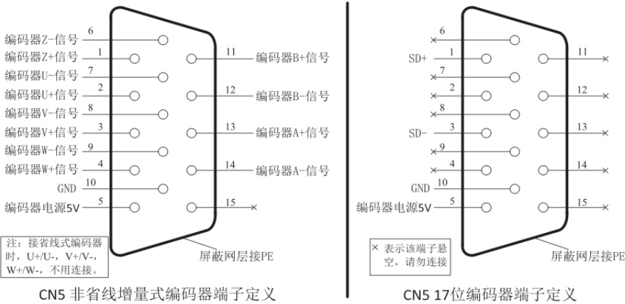
图 3-6 CN5 端子引脚分布
