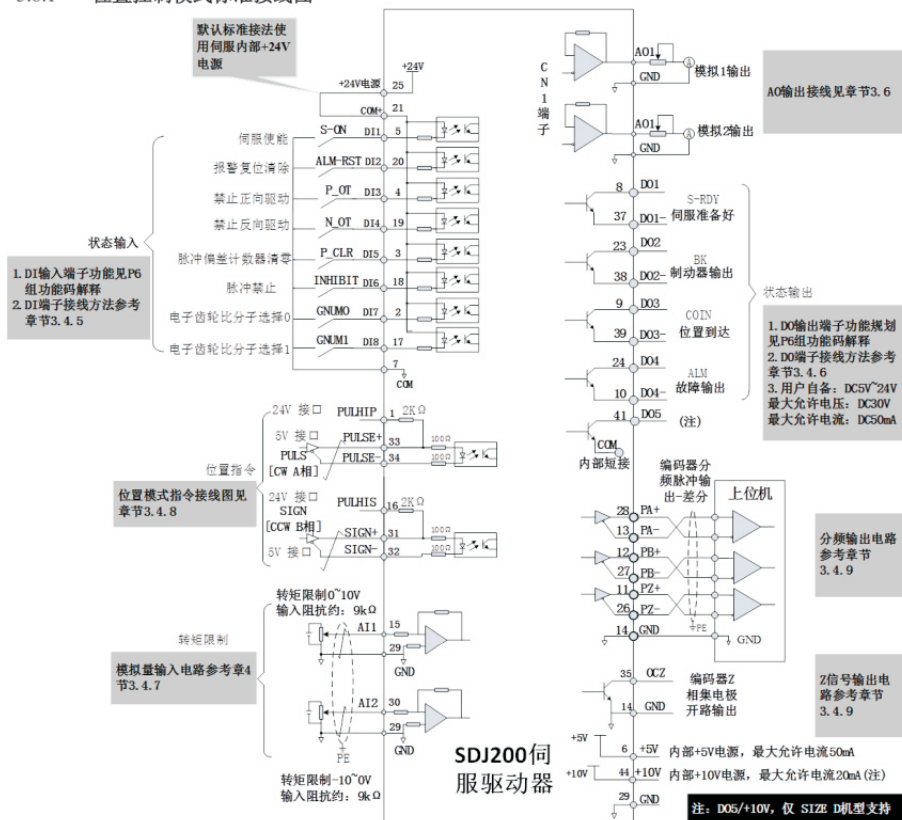
图 3-24 位置模式标准控制电路接线图
