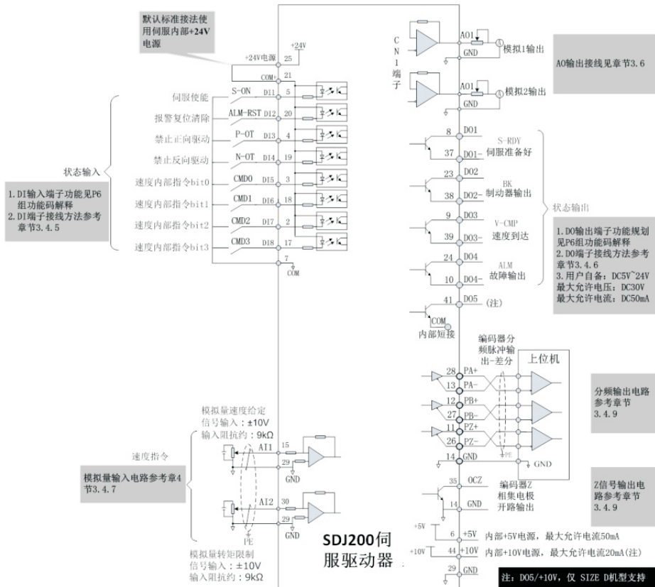
图 3-25 速度模式标准控制电路接线图
