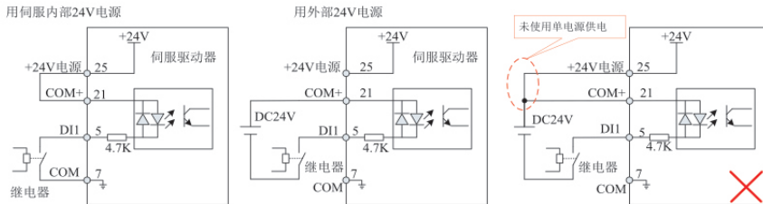
图 3-8 上级装置为继电器输出时的数字输入端子接线
