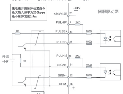
图 3-15(b) 集电极开路方式输入脉冲指令接线图（使用外部电源及外接限流电阻）
