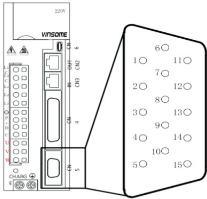
图 3-4 CN5 端子位置
