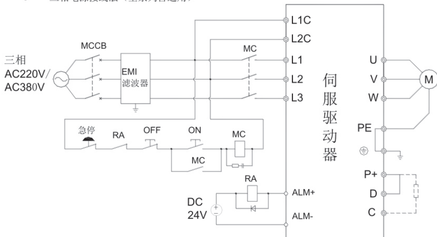
图3-2 三相电源接线图
