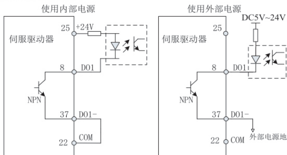
图 3-11 (a) 上级装置为光耦输入时的数字输出端子正确接线
