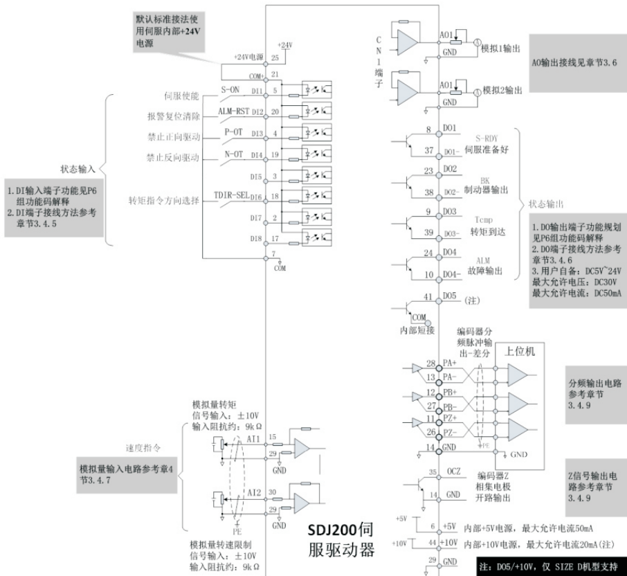
图 3-26 转矩模式标准控制电路接线图
