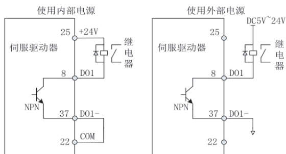
图 3-10(a) 上级装置为继电器输入时的 DO 端子正确接线
