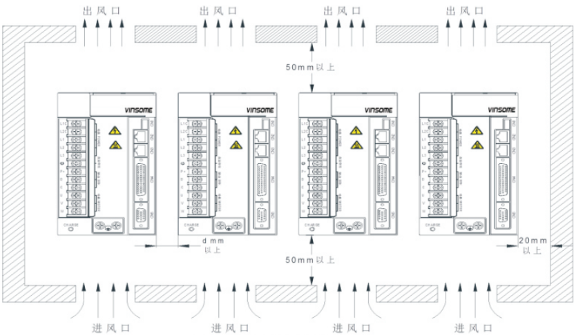
图 2-1 伺服驱动器安装空间
