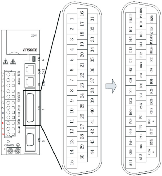
图 3-7 驱动器控制回路端子位置及引脚分配图
