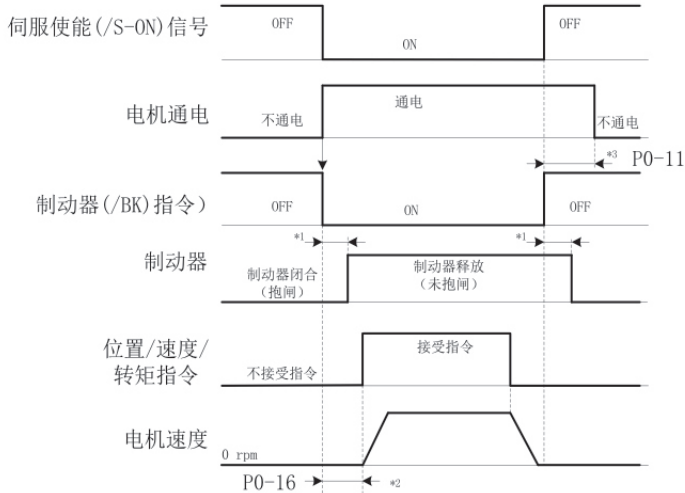
图 3-21 保持制动器释放和闭合延迟时间
