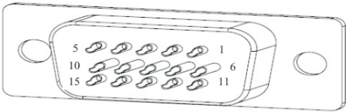
图 3-5 CN5 端子焊接引脚分布
