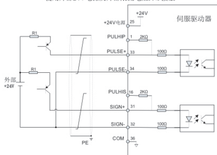
图 3-15(b) 集电极开路方式输入脉冲指令接线图（使用外部电源及外接限流电阻）
