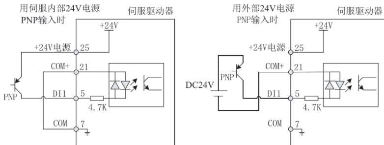
图 3-9(b) 上级装置为集电极 PNP 开路输出时的数字输入端子接线
