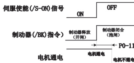
图 3-22 伺服取消使能时制动器动作时序
