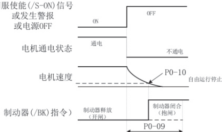
图 3-23 伺服电机旋转时的制动器动作
