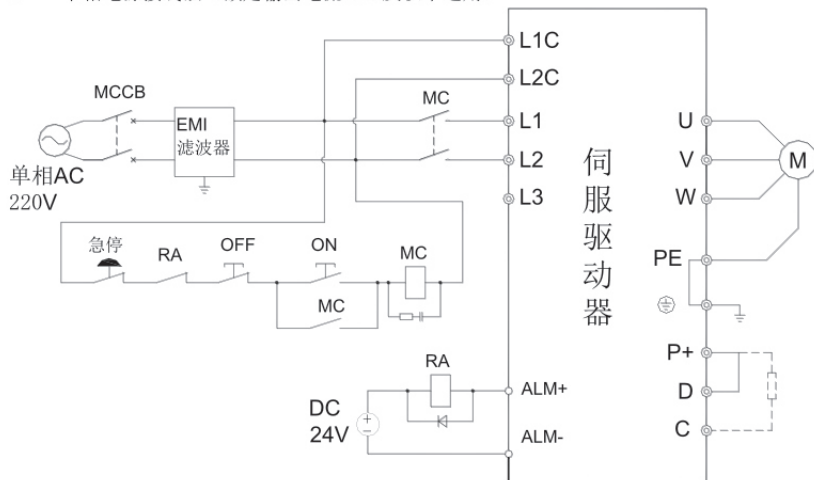
图3-1 单相电源接线图
