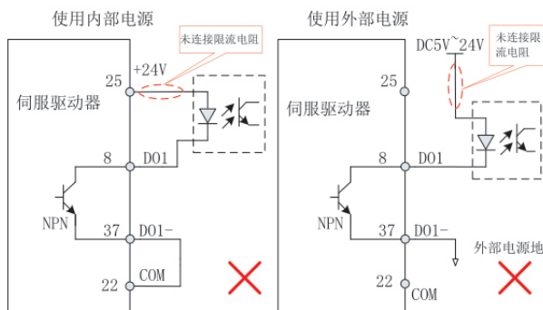
图 3-11 (b) 上级装置为光耦输入时的数字输出端子错误接线
