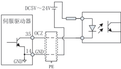
图 3-18 OCZ 端子配线图
