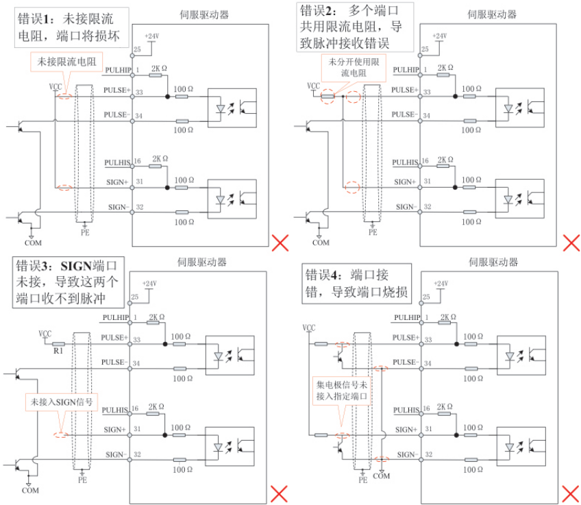
图 3-16 4 种典型错误接线
