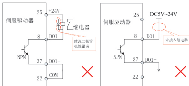
图 3-10(b) 上级装置为继电器输入时的 DO 端子错误接线
