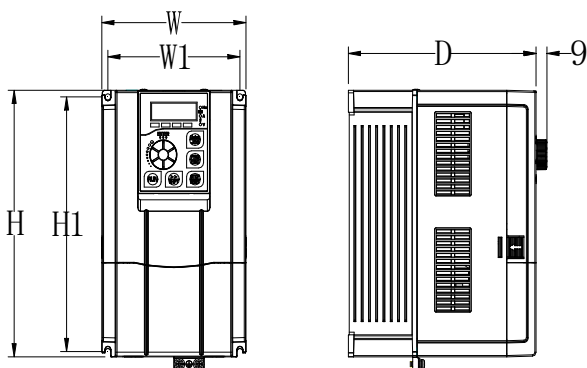
图 2-4. 380V 15KW 以下塑胶外形尺寸及安装尺寸示意图
