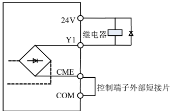
内部供电接线图
