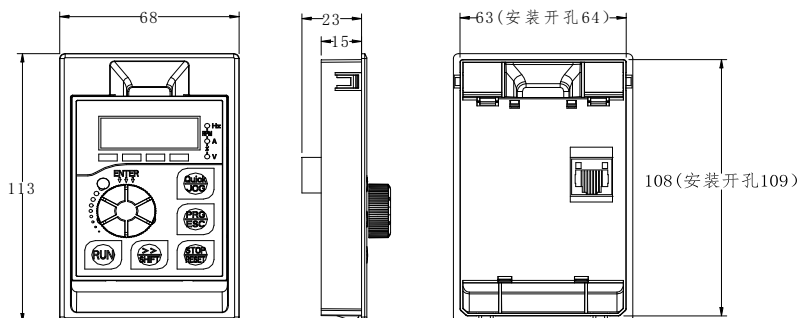
图 2-8.1 小外引键盘带托盘安装尺寸图 (4T:380V 37kW以下标配小外引键盘)
