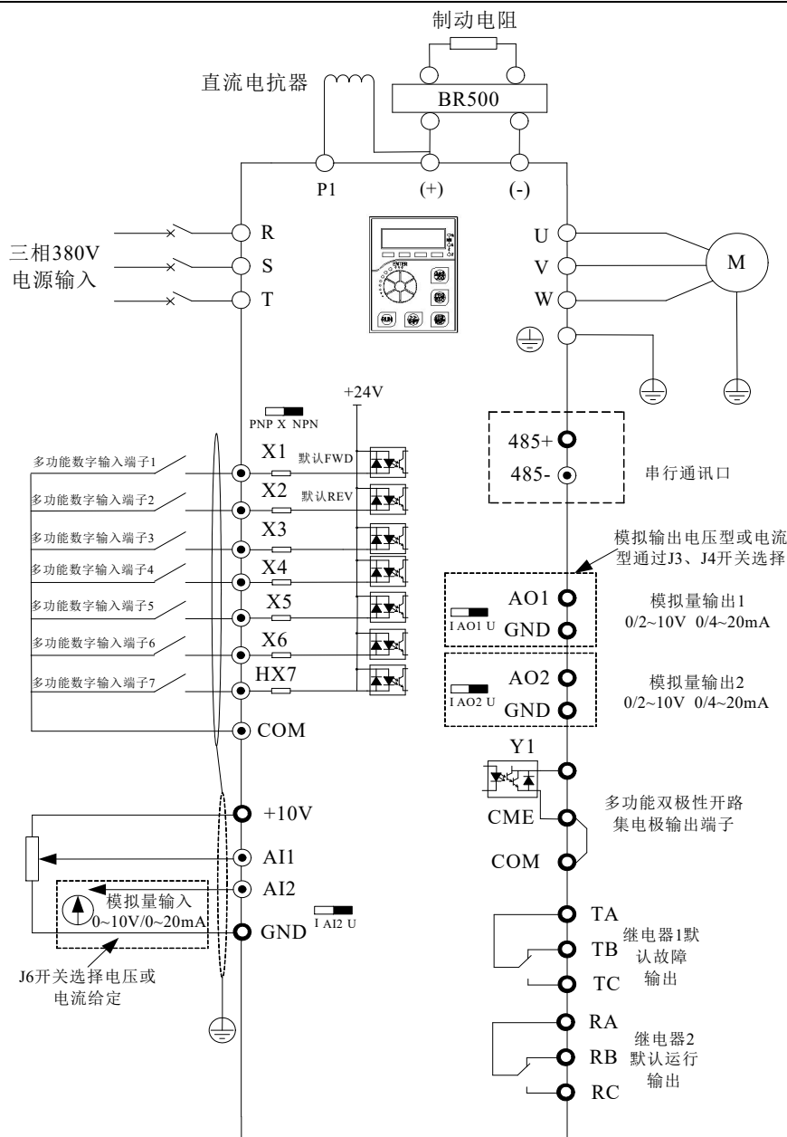
图 3-4. 75Kw (4T:380V 75 Kw) 及以上三相变频器
