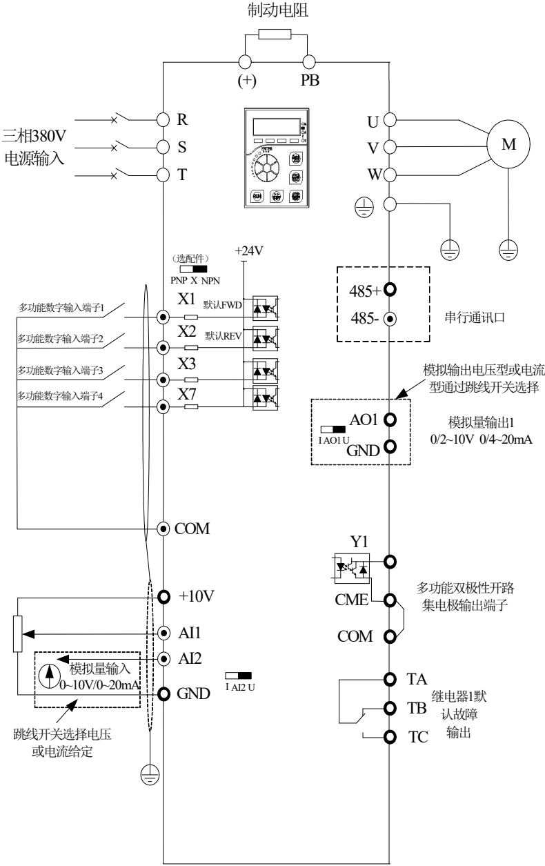
图3-1.2.2kW (4T:380V 2.2 kW) 以下三相变频器接线图
