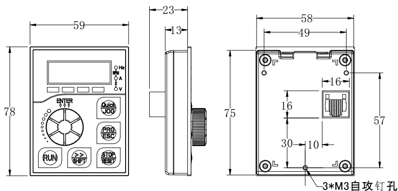
图 2-9.1 小外引键盘不带托盘安装尺寸图 (4T:380V 37kW以下标配小外引键盘)
