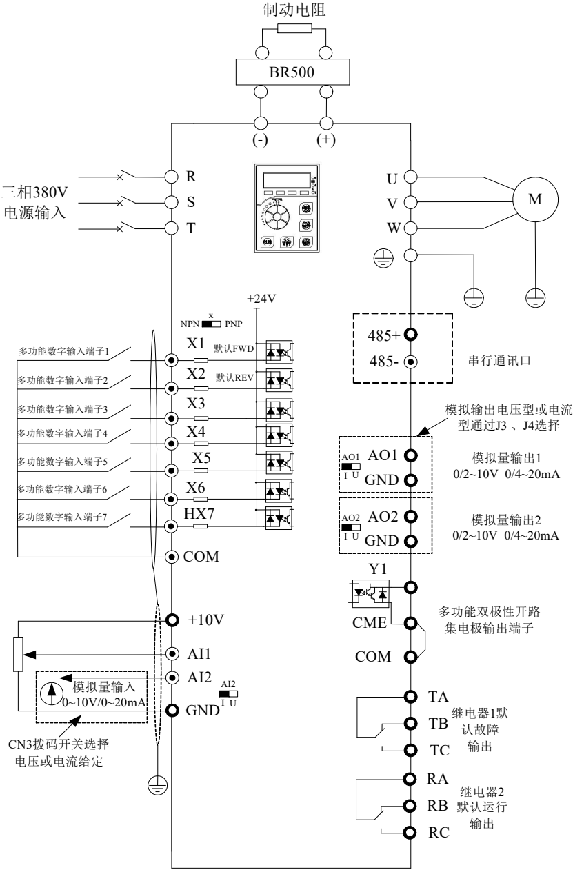
图 3-3.30 ~ 55Kw (4T:380V 30 ~ 55 Kw) 三相变频器不带制动单元功能接线图
