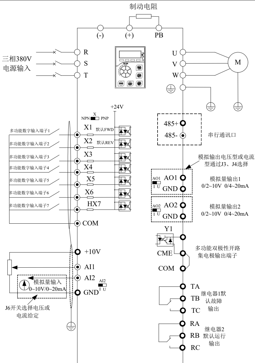
图 3-2. 4.0 ~ 22kW (4T:380V 4.0 ~ 22kW) 三相变频器接线图
