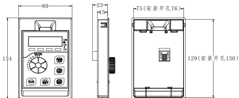
图 2-8.2 大外引键盘带托盘安装尺寸图 (4T:380V 45kW以上标配大外引键盘)
