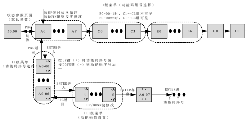
图 4-2. 三级菜单操作流程图
