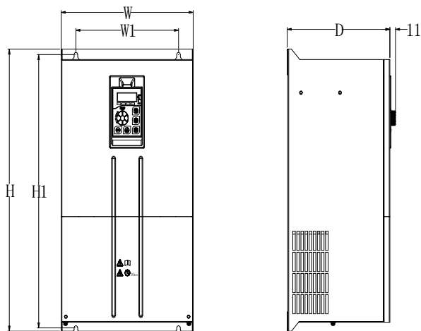
图 2-5. 380V 18.5~132KW 钣金机箱外形尺寸及安装尺寸示意图
